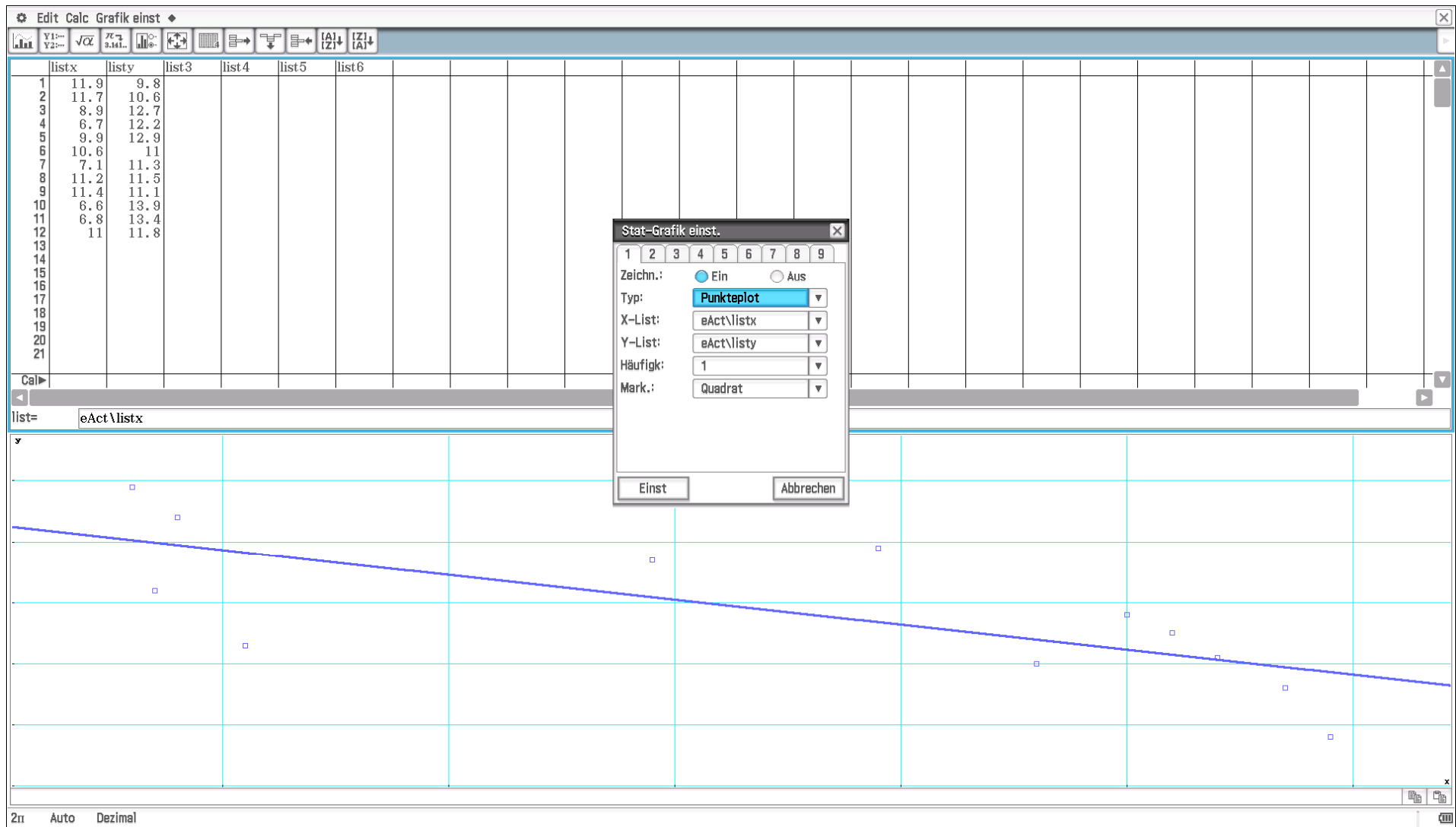
Aufg. A5: a) Streuungsdiagramm (Scatterplot) und c) Regressionsgerade
