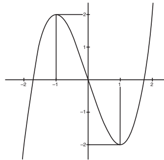
Übersichtstabelle und Grafik für y = x^3 - 3x (Die rechte Grafik dient nur als Referenz.)
